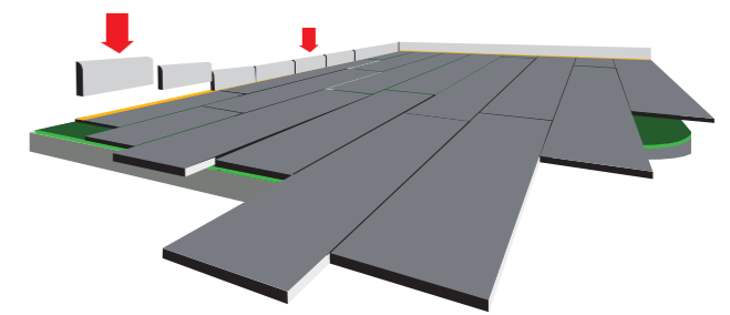
FASE 10. Posa diretta del battiscopa sul distaccante per battiscopa D-Stick.
